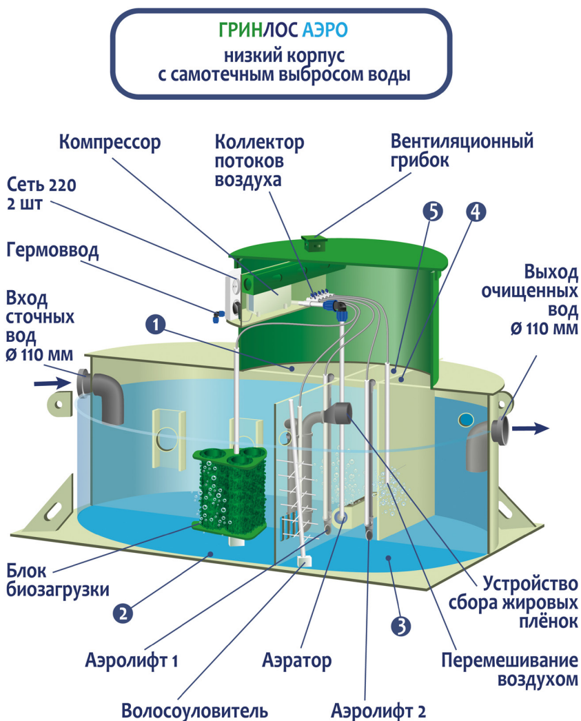
Рисунок 8. Схема Изделия ГРИНЛОС АЭРО с самотечным сбросом (низкий корпус).
